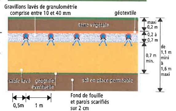
COUPE TRANSVERSALE
